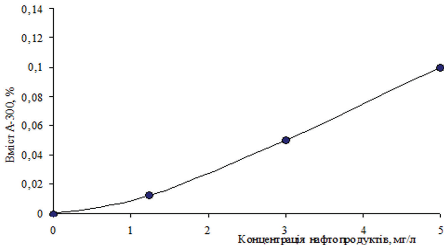
Рис. 2. Залежність залишкового вмісту нафтопродуктів у питній воді від їх початкової концентрації після очищення води «А-300».
