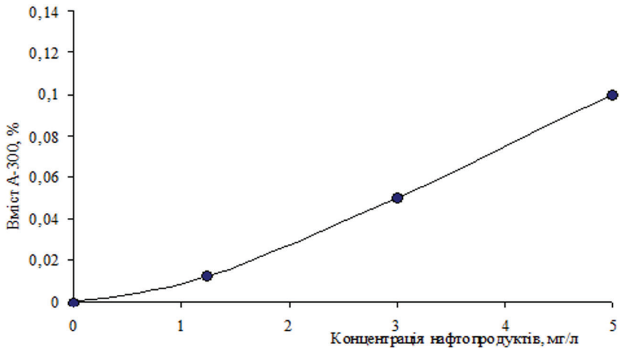
Рис. 1. Залежність кількості „А-300”, необхідної для очищення забрудненої нафтопродуктами питної води, від їх концентрації.
